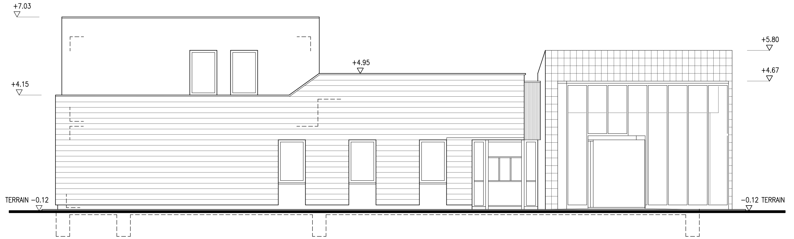
OSTANSICHT
