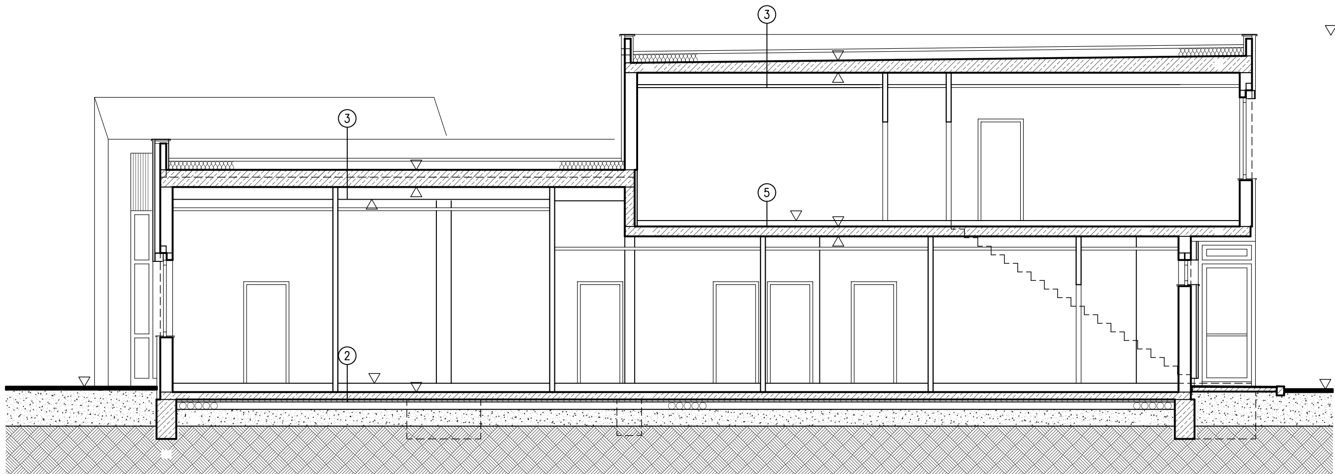
SCHNITT 1 -- 1
