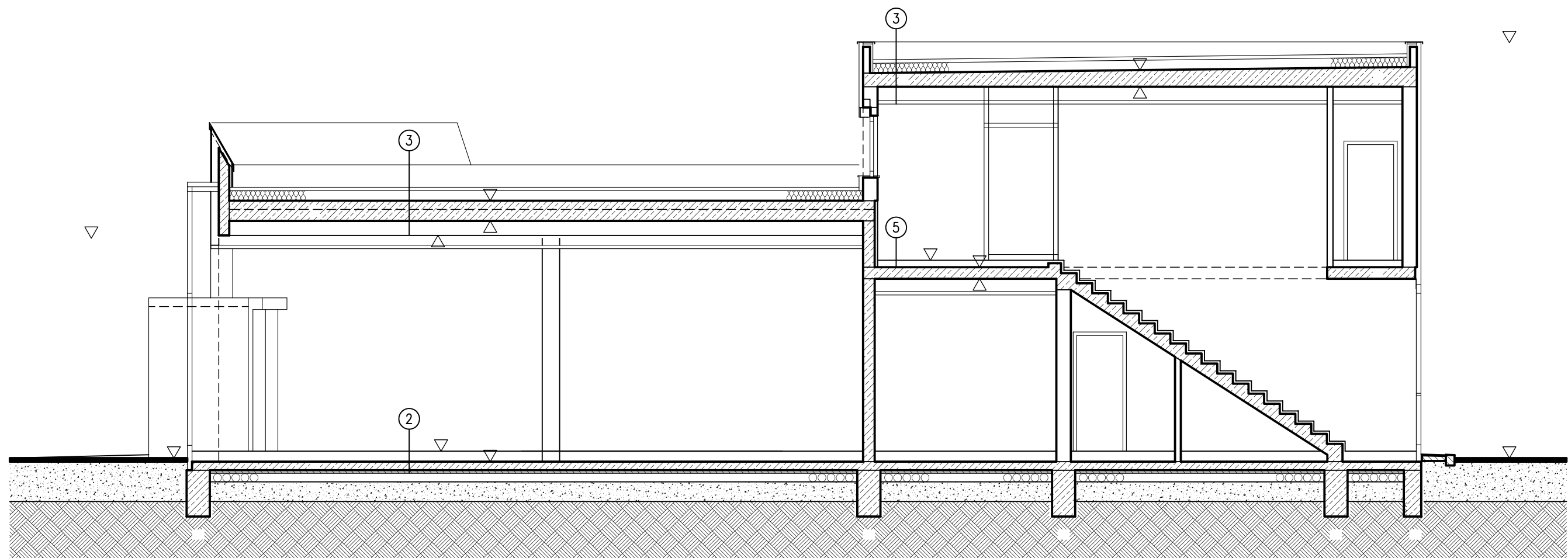
SCHNITT 2 -- 2
