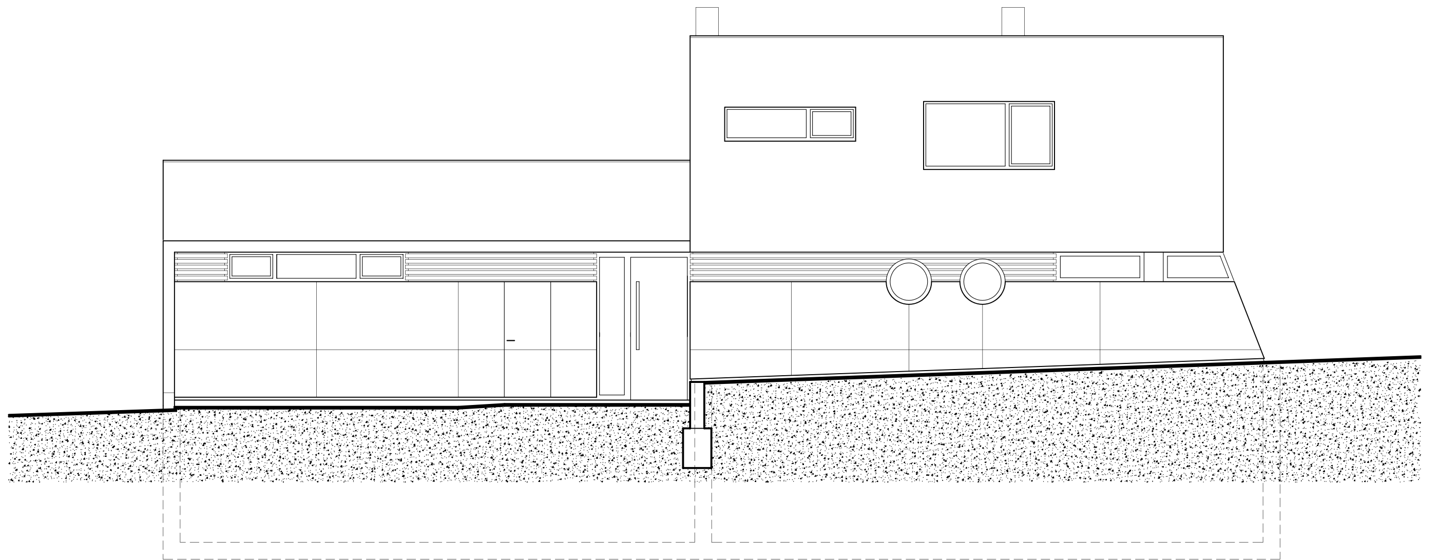
NORDANSICHT
