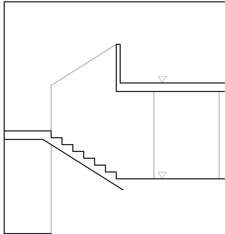
SCHNITT C-C
