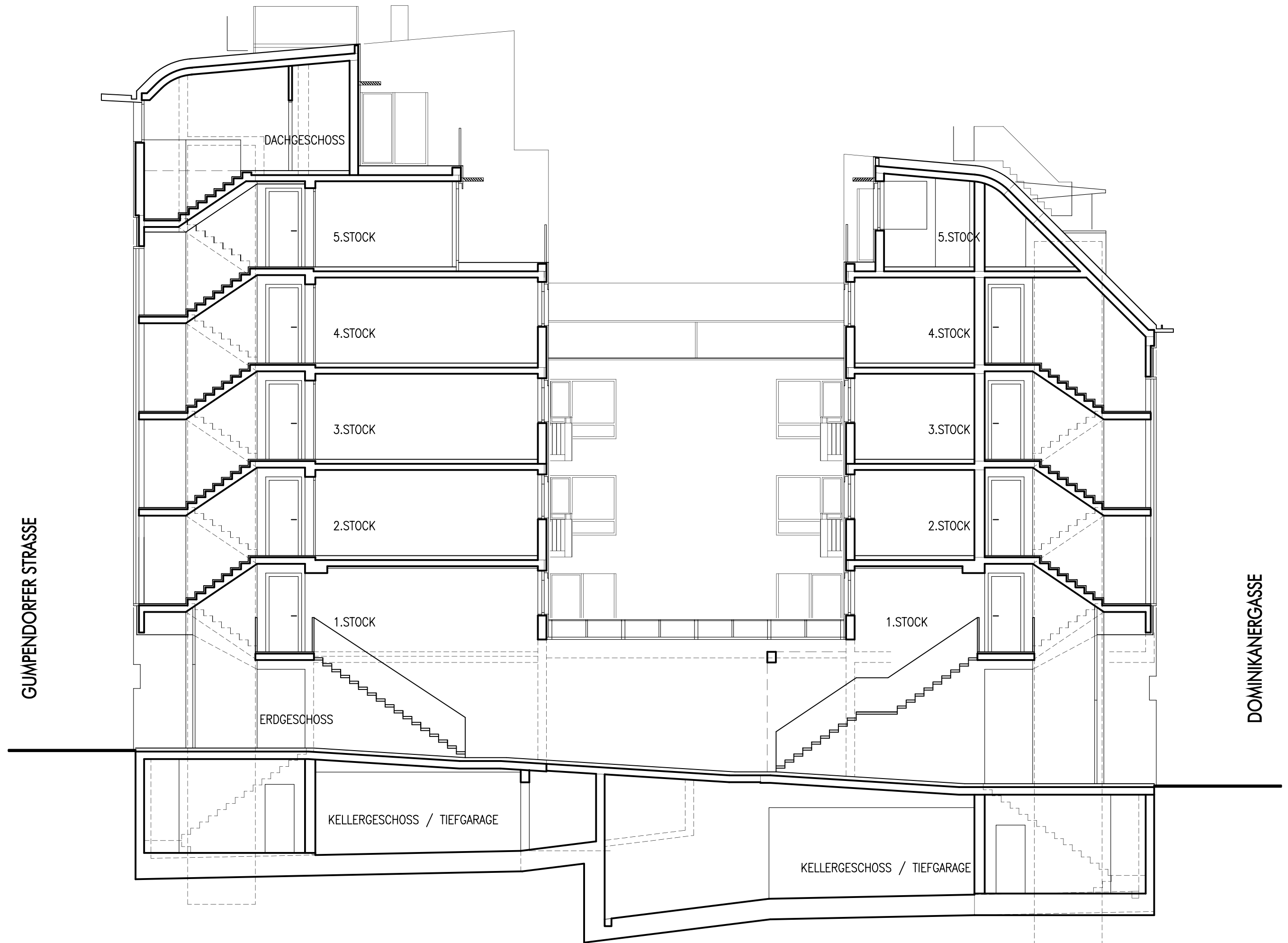
SCHNITT 2 - 2
