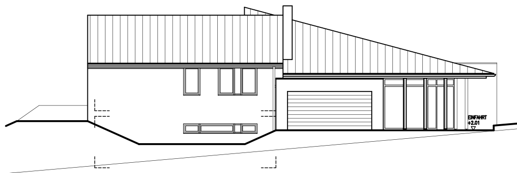
STRASSENANSICHT OSTEN
