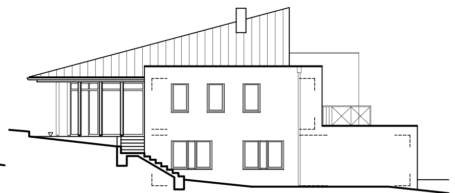
SEITENANSICHT WESTEN
