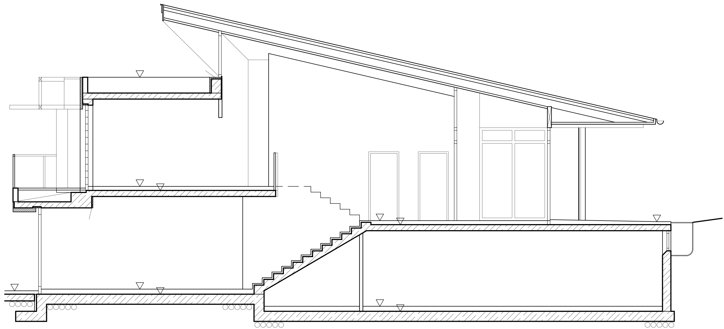
SCHNITT 1 -- 1
