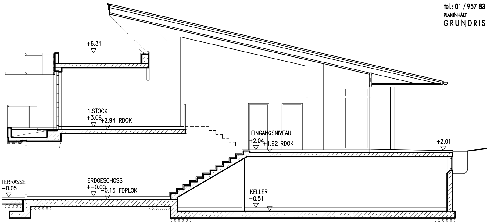
SCHNITT 1 -- 1
