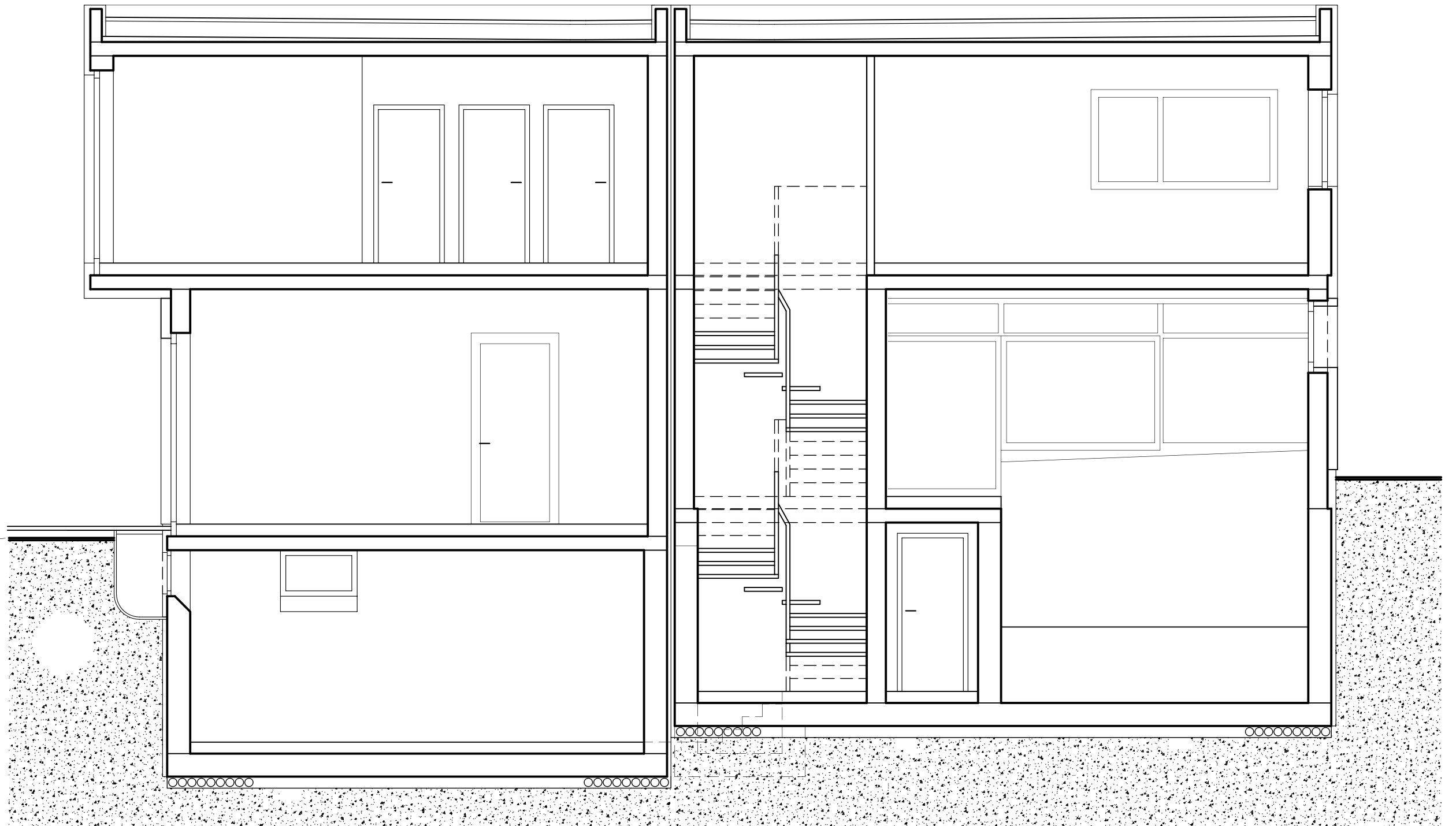
SCHNITT 1--1
