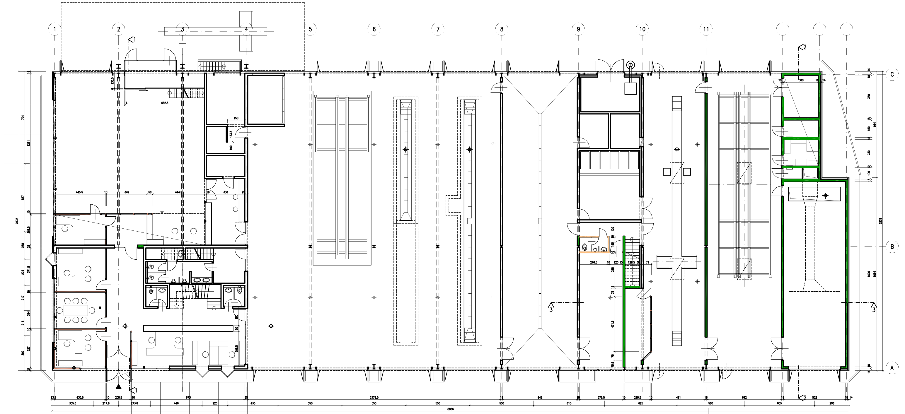
ERDGESCHOSSGRUNDRISS
